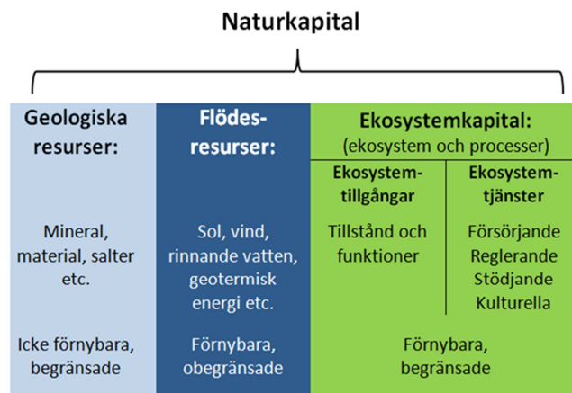
Figur 1. Naturkapitalets komponenter 31
